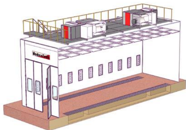
Технические характеристики серии МТ 2 3007
